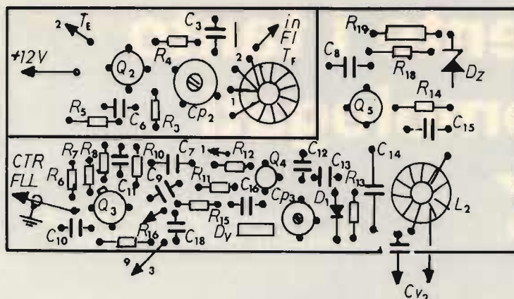
MIXER - VFO e BUFFER: lato componenti, 1:1.
