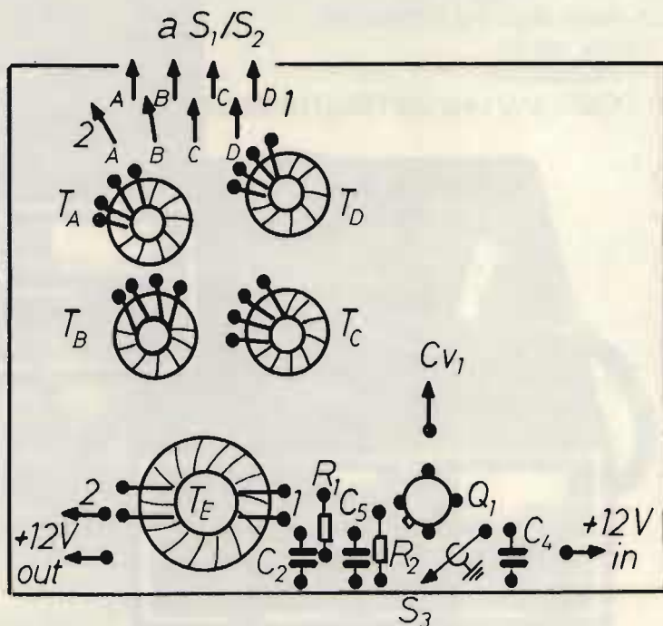
Preselettore: lato componenti, 1:1.
